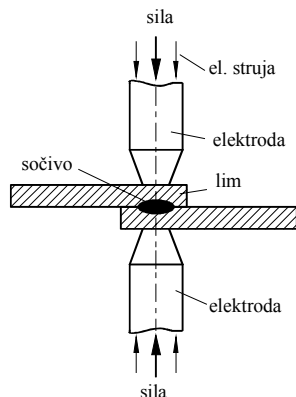
Slika 1. Shema tačkastog zavarivanja
