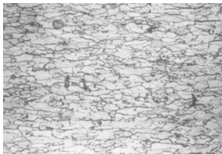
O.M. - Sitnozrna, pretežno feritna struktura sa neznatnim učešćem perlita (200×)
