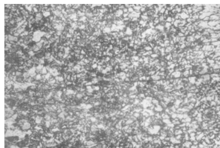
ZUT - usitnjena, normalizovana feritna struktura sa neznatnim učešćem perlita (200×)
