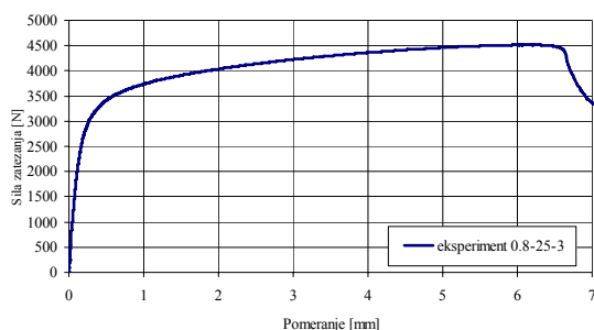
Slika 8. Dijagram sile - pomeranje; zatezanje tačkasto zavarene epruvete debljine 0.8 mm i širine 25 mm
