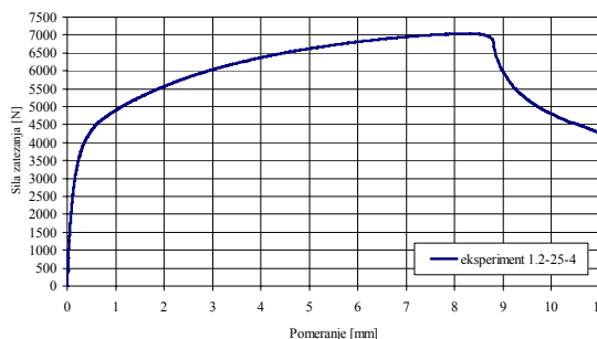
Slika 9. Dijagram sile - pomeranje; zatezanje tačkasto zavarene epruvete debljine 1.2 mm i širine 25 mm
